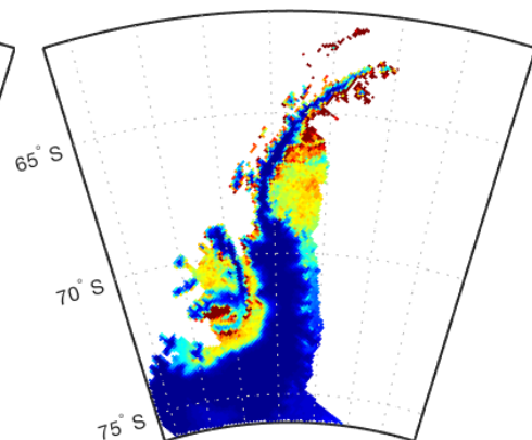
(d) MAR SD melt
